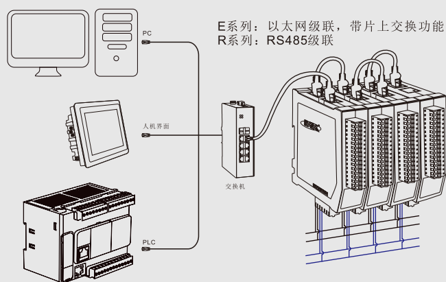
CK模块通过RS485级联接口设备组网连接示意图
