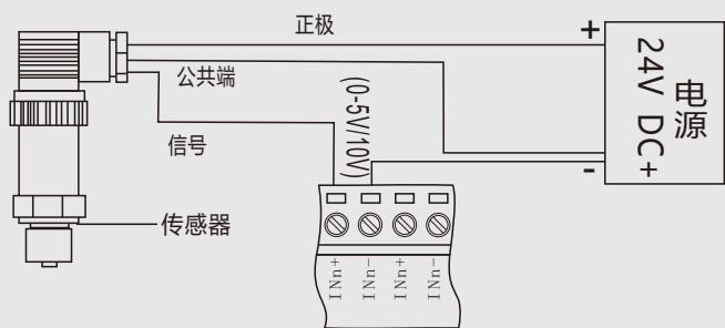
三线制电压输出接线图
