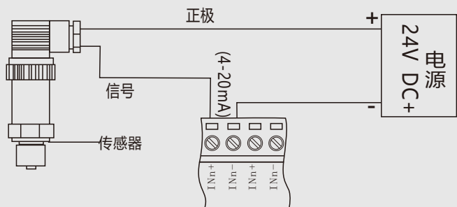
两线制电流输出接线图
